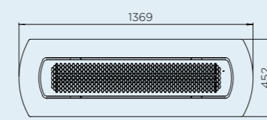
PLAFONDINBOUWFRAME 2000W & 4000W
